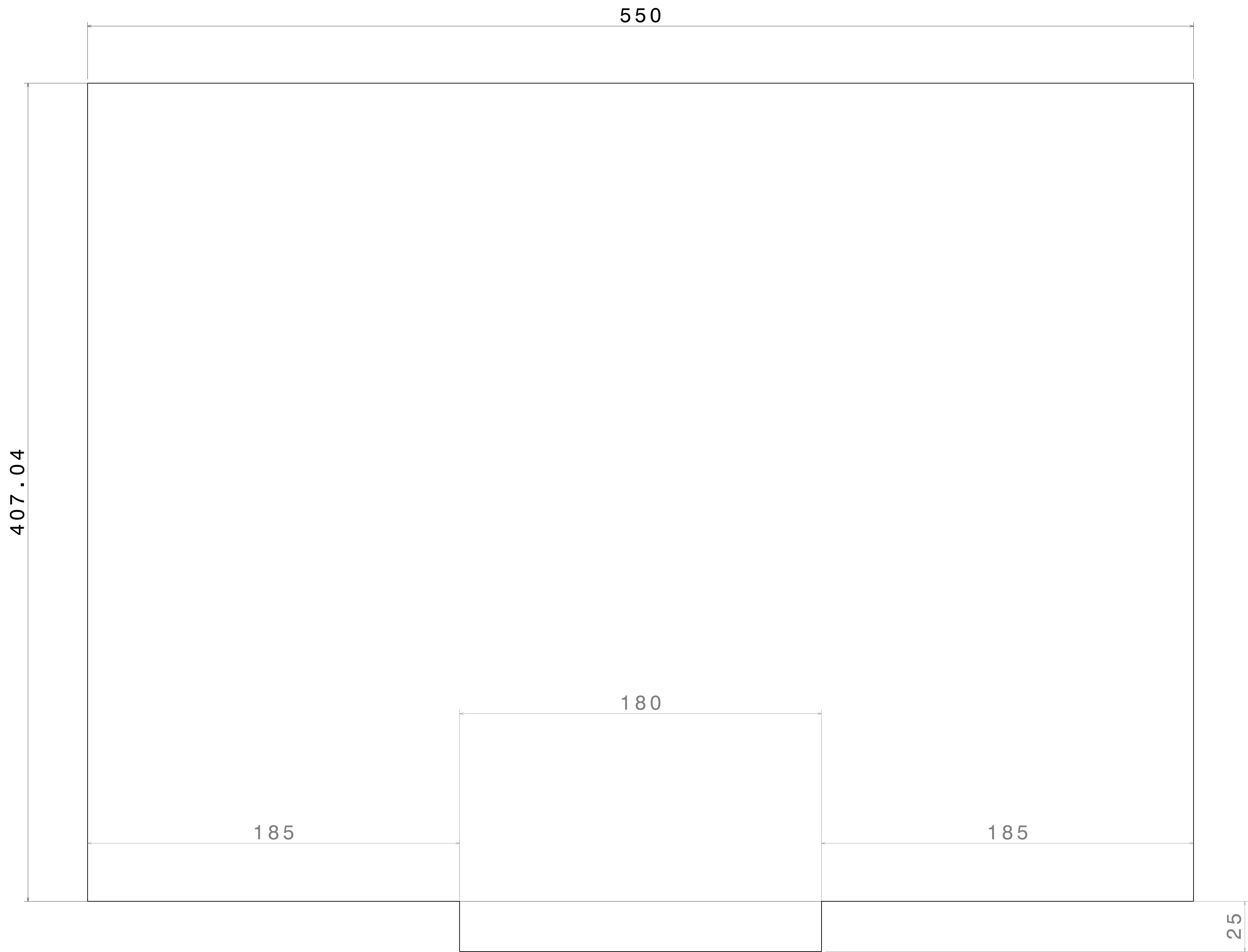
Vue de face Echelle : 1:1
