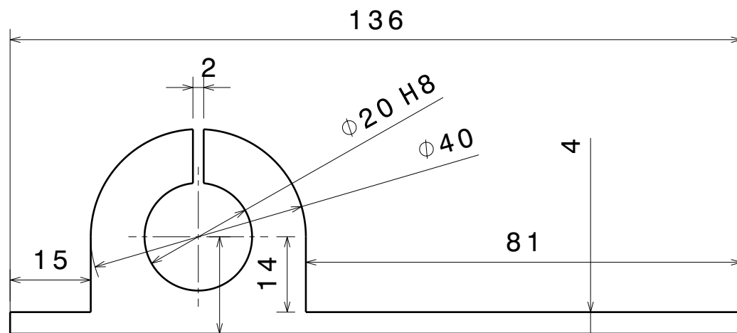
Vue de dessous Echelle : 1:1
