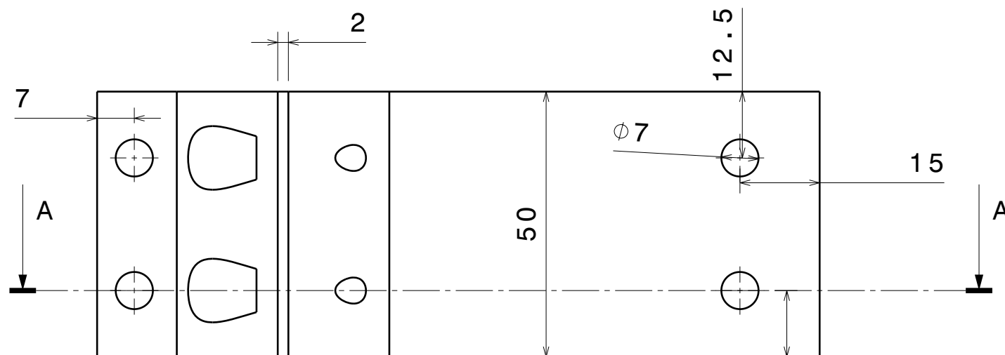
Vue de face Echelle : 1:1
