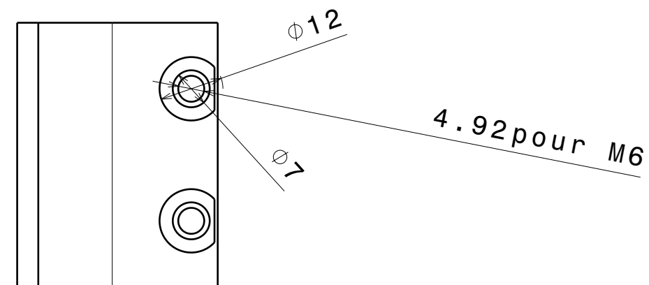
Vue de gauche Echelle : 1:1
