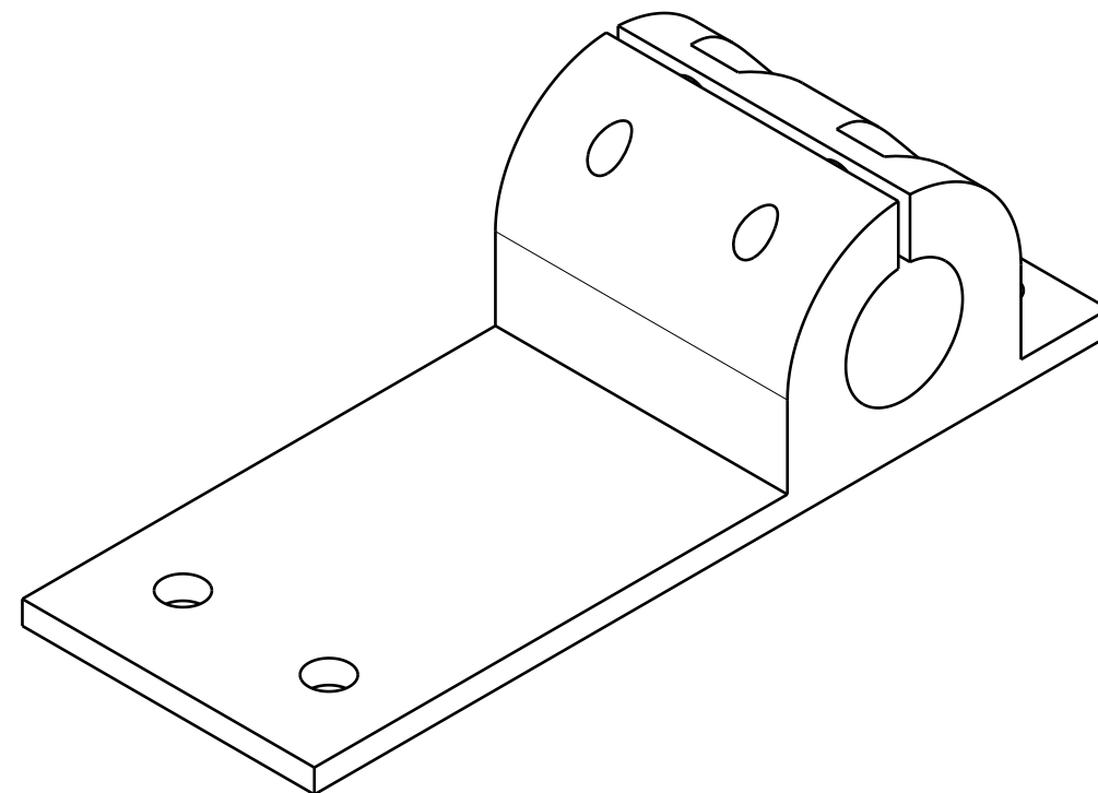
Vue isométrique Echelle : 1:1
